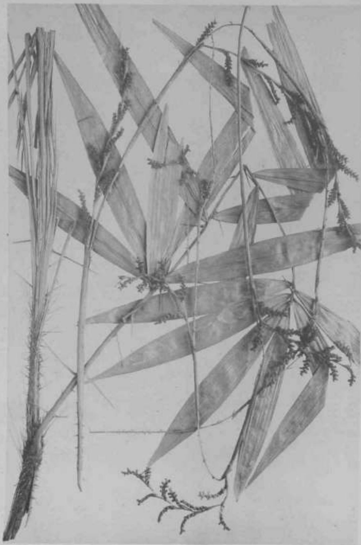
CALAMUS DRACUNCULIFOLIUS.
